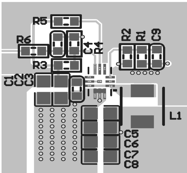
Top Layer
